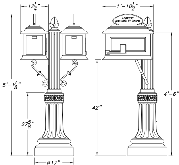
SCALE: 1/2"=1'-0" CL-17-2-SSR
